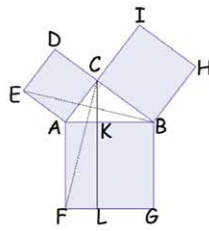
圖 2-2 歐幾里得的畢氏定理證明
